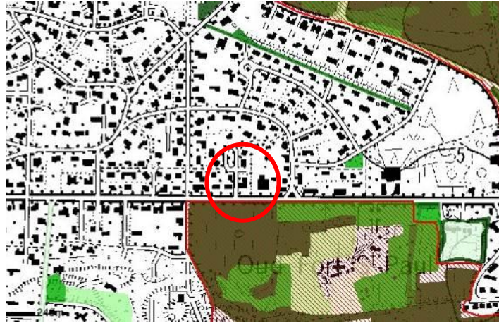
Biologische waarderingskaart
