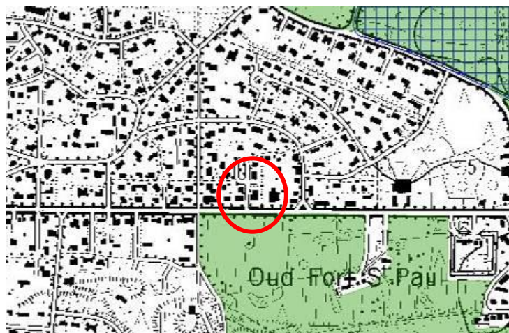
Habitatrictlijngebied
